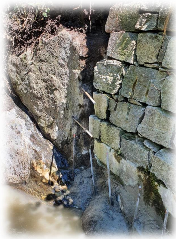
Sopra: Arbedo - Opere di rinforzo al muro di contenimento.
